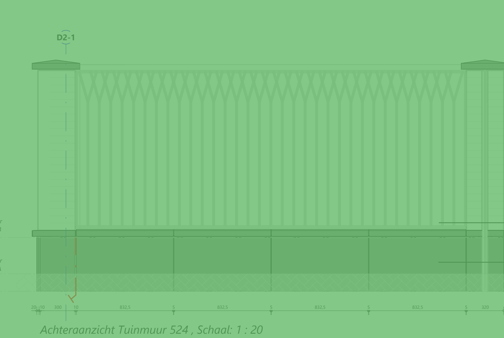
Achteraanzicht Tuinmuur 524, Schaal: 1 : 20
